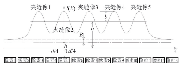
图7 红外狭缝靶标的采样模型
