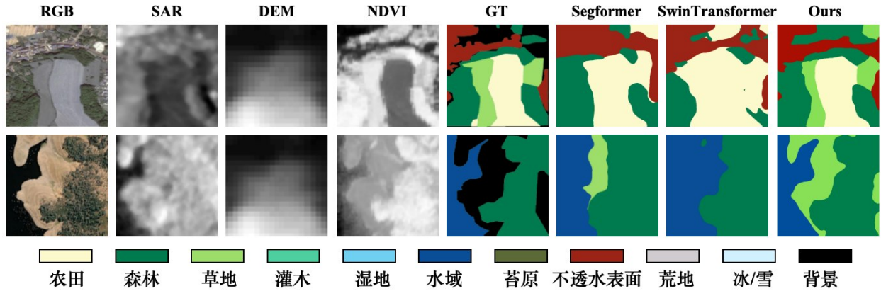
图3 Globe230k数据集的可视化结果
