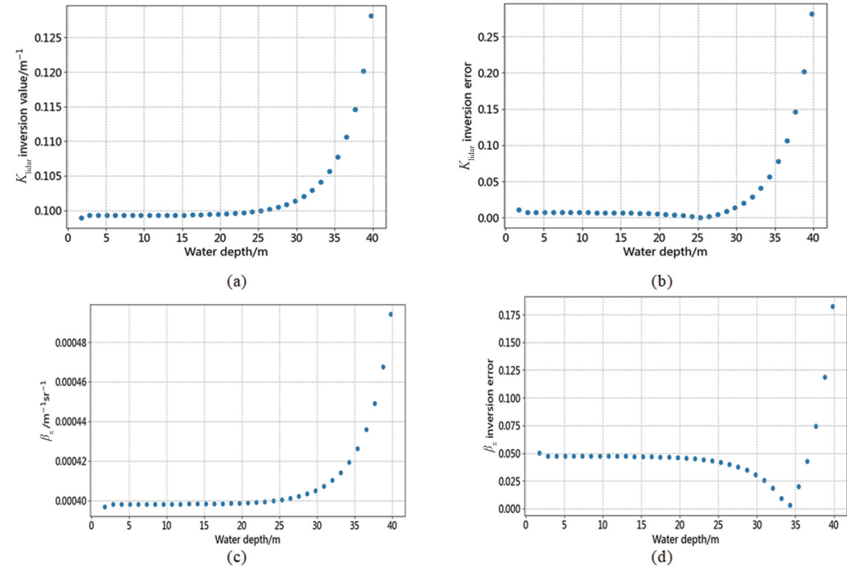
图9 Fernald法水体光学参数反演误差分析:(a) K_{\text{lidar}} 反演值;(b) K_{\text{lidar}} 反演误差;(c) \beta_\pi 反演值;(d) \beta_\pi 反演误差 Fig. 9 Error analysis of inversion of water optical parameters by Fernald method: (a) K_{\text{lidar}} inversion value; (b) K_{\text{lidar}} inversion error; (c) \beta_\pi inversion value; (d) \beta_\pi inversion error
