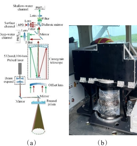
图1 海洋剖面激光雷达系统:(a)原理图;(b)实物图
