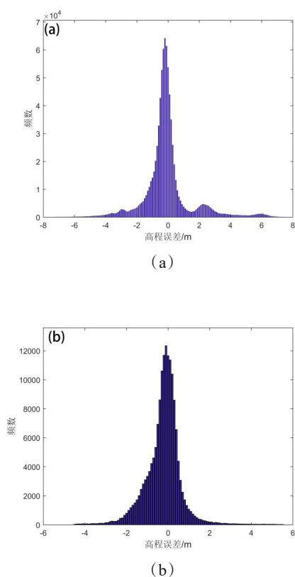
图4 陆碳监测卫星激光测高数据筛选前后精度验证结果: (a)原始数据;(b)筛选后数据
