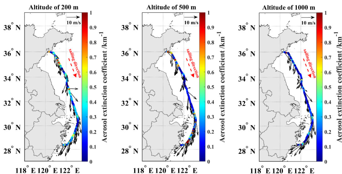
图12 大气多参数探测激光雷达2024年8月6日19:00至12日06:00观测海上不同高度(200 m、500 m、1 000 m)气溶胶消光系数、风速、风向分布图
