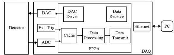
Fig. 8 Test module diagram 图8 测试模块结构框图
