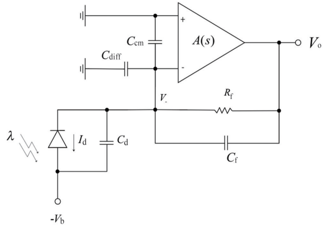
Fig. 2 The transimpedance circuit model 图2 跨阻电路模型
