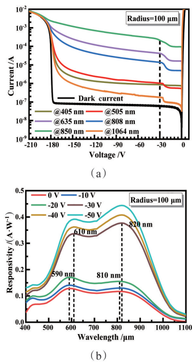
图 4 SACM APD 的 I - V 光电流特性及光谱响应:(a) 100\text{ }\mu\text{m} SACM APD 在不同波长下的 I - V 光电流;(b) 100\text{ }\mu\text{m} SACM APD 在不同偏压下的光谱响应
