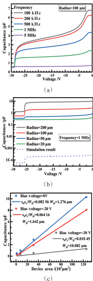
图5 SACM APD的 C - V 特性。(a)不同频率下100 \mu\text{m} SACM APD的 C - V 特性;(b)1 MHz下不同光敏面半径SACM APD的 C - V 特性(虚线为半径100 \mu\text{m} 器件在1 MHz频率下电容仿真曲线);(c)不同尺寸器件在0 V、-20 V、-30 V偏压下的电容值及电容与器件光敏面面积拟合关系
