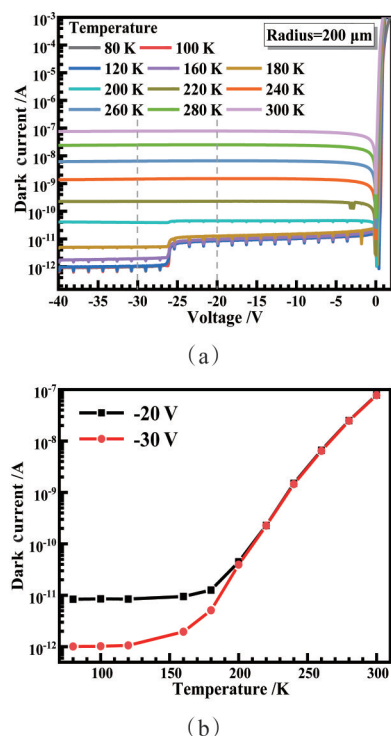
图6 SACM APD 的温度特性:(a)不同温度下 200 \mu\text{m} SACM APD 的暗电流特性;(b)-20 V 和-30 V 偏压下器件暗电流随温度的变化关系
