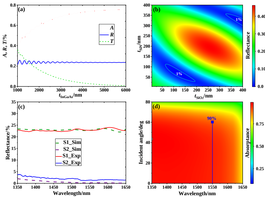
图4 光学仿真结果和实验结果:(a) \lambda=1\,550\,\text{nm} 时,无减反层器件吸收率( A )、反射率( R )、透射率( T )随吸收层厚度 t_{\text{InGaAs}} 的变化关系图;(b) t_{\text{InGaAs}}=4\,050\,\text{nm} , \lambda=1\,550\,\text{nm} 时,器件的反射率随减反层 \text{SiO}_2 和 \text{SiN} 厚度的变化关系图;(c)器件反射谱的计算与实验结果对比图,S1为沉积了 \text{SiO}_2/\text{SiN} 减反层的样品,S2为未沉积减反层的样品;(d) t_{\text{InGaAs}}=4\,050\,\text{nm} , t_{\text{SiO}_2}=140\,\text{nm} , t_{\text{SiN}}=60\,\text{nm} 时,器件吸收率随激光波长和入射角度变化图
