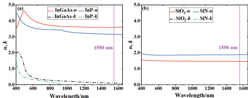
图3 材料光学参数测试:(a)外延InP、 \text{In}_{0.53}\text{Ga}_{0.47}\text{As} 薄膜的光学参数(折射率 n 和消光系数 k )随波长的变化关系图;(b)减反层 \text{SiO}_2 和SiN薄膜的光学参数随波长的变化关系图
