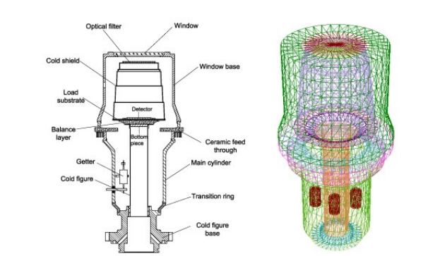
图 8 实验杜瓦 1 的结构和计算模型 Fig. 8 Structure and computational model of experimental Dewar 1
