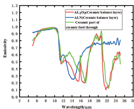
图6 非灰体发射率
