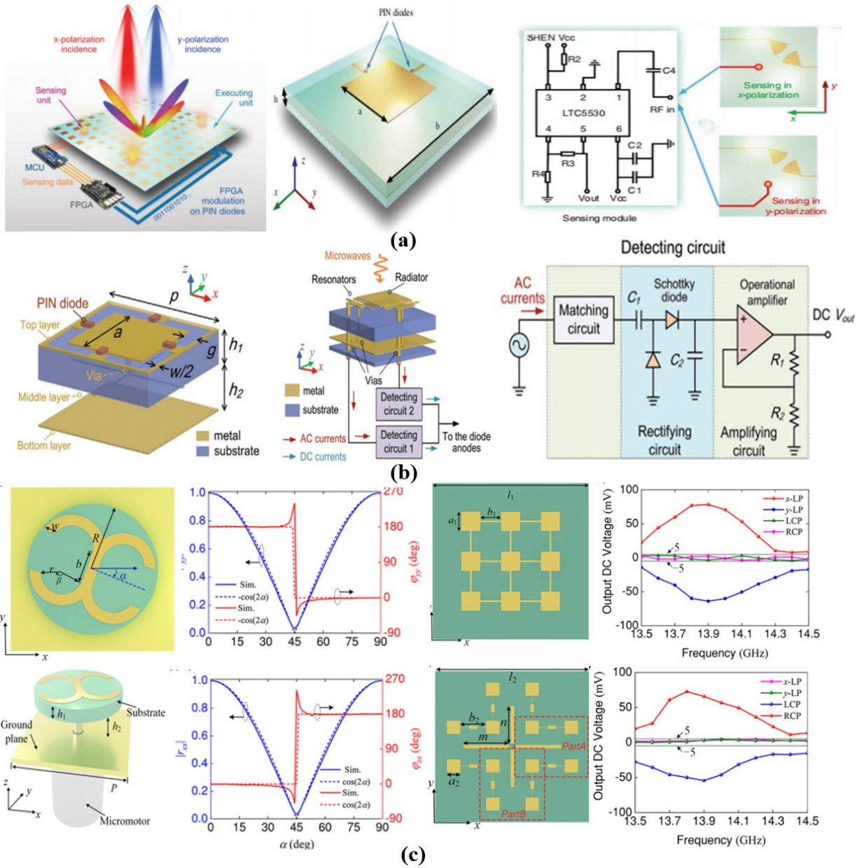
图9 (a)所提出的智能传感超表面的原理图,设计的用于感知和执行目标的数字编码元件,x和y极化传感单元的传感机制 [100] ; (b)吸收超表面单元、传感天线和以下检测电路的三维视图、在仿真中的检测电路的原理图模型 [101] ; (c)超表面单元,反射系数 r_{xx} 和 r_{yy} 的幅值和相位作为参数 \alpha 在14 GHz时的函数,入射极化检测的传感模块及测量的输出直流电压 [102]
